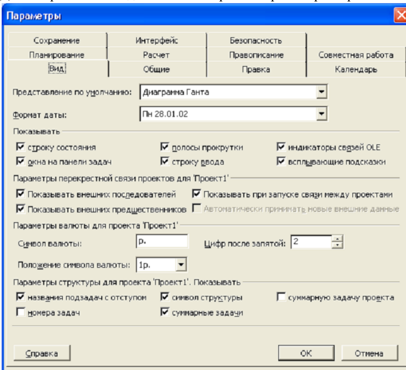
Рис. 3 – Вкладка «Параметры»
